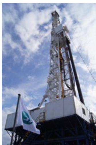
掘削中の様子
